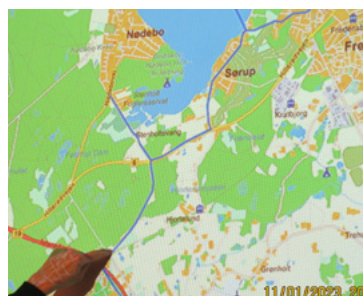
En mulig transmissions-ledning for fjernvarme (blå linie) fra Hillerød Øst til Nødebo og Sørup, som Hillerød Forsyning viste os d. 11. januar.
